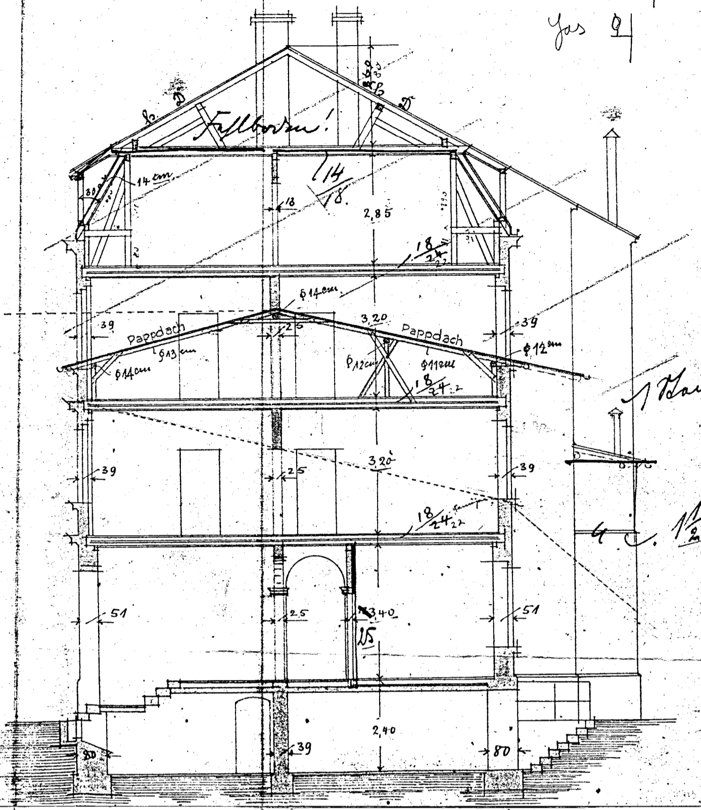
Schnitt A-B.
